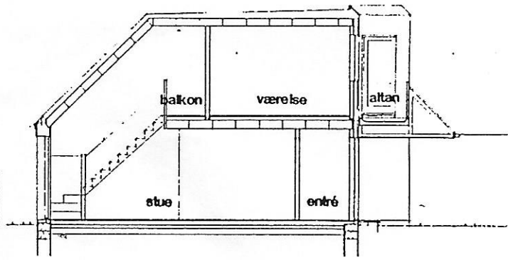
SNIT 1:100
