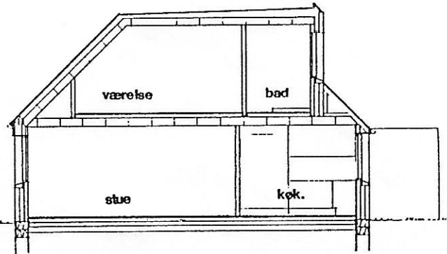
SNIT 1:100
