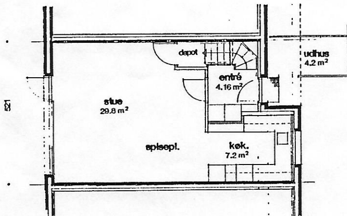
STUEPLAN 1:100
